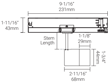
Luminaire
