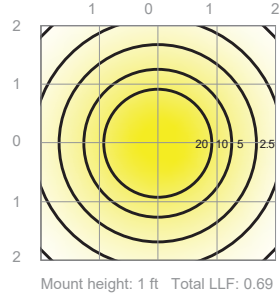
Isofootcandle Plot
